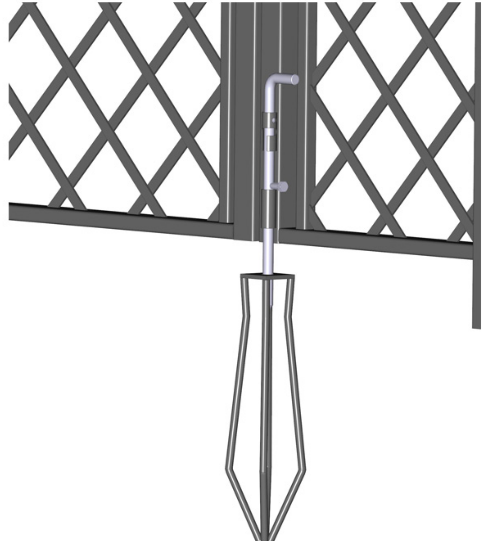
mittiger Anker (geschlossen)
